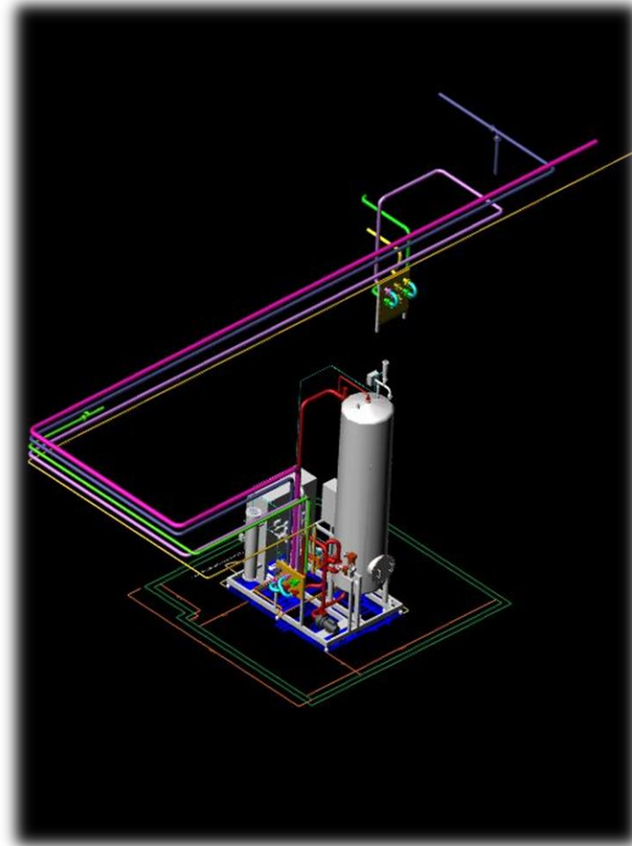
Modelo 3D
